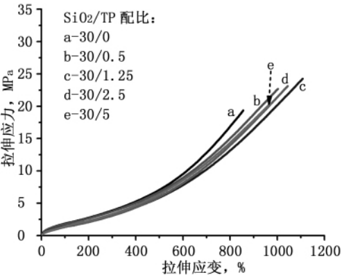
图 5 TP 改性 SiO 2 /NRL 复合材料应力应变曲线
