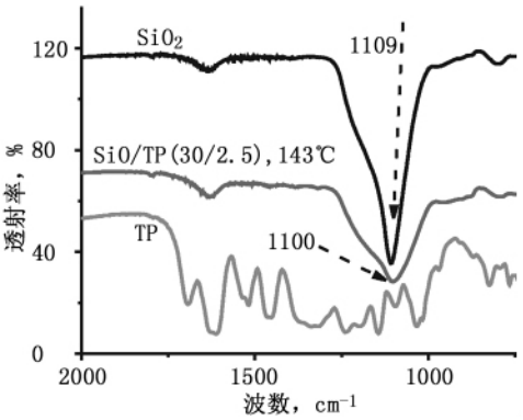
图 3 TP,SiO 2 及其模型化合物的红外光谱
